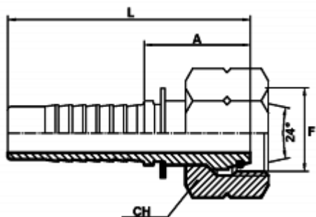
Накрайник DKOL с O-пръстен конус 24° по DIN 3865
