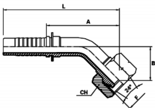
Накрайник DKOL с O-пръстен конус 24° по DIN 3865 ъгъл 45°
